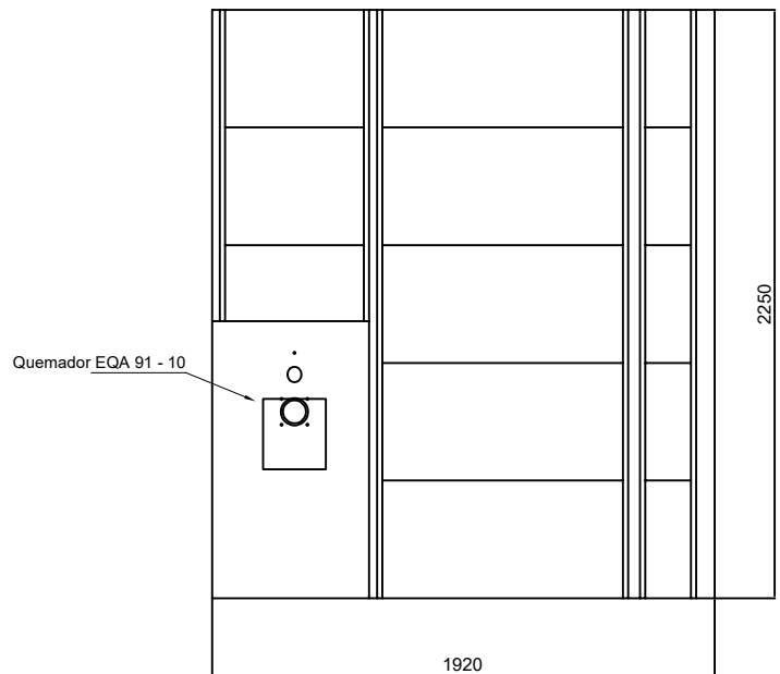
VISTA LATERAL QUEMADOR
