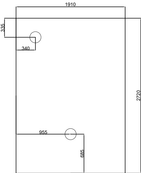
VISTA SUPERIOR
